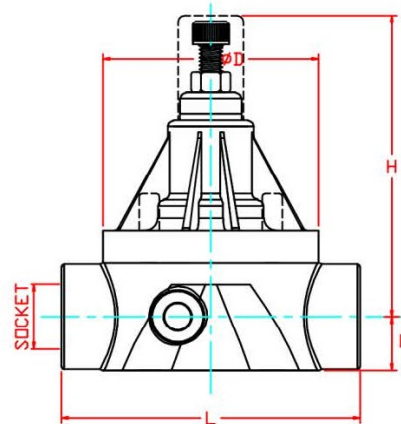
Socket
