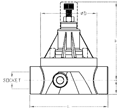
Socket
